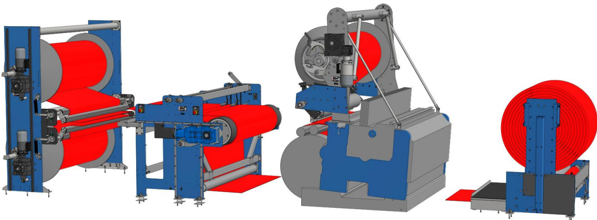
Kettbaumgestell, Lieferwerk, Spezialwebmaschine mit Kettbaum in Hochlage, Dockenwickler
