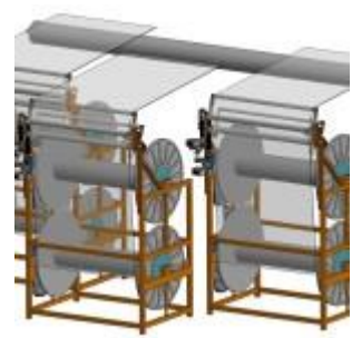
Fadenzuführsystem für Kettenwirkmaschinen
